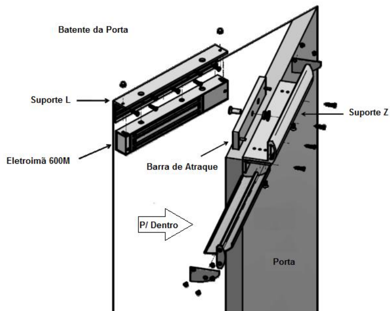
Figura 1: Vista expandida
