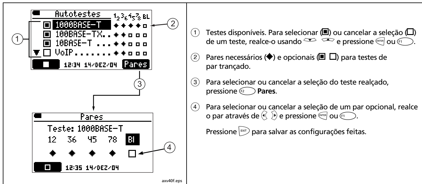
Figura 5. Telas de configuração de Autoteste
