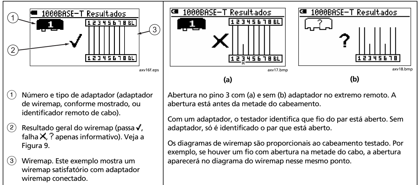
Figura 10. Exibição típica de wiremap
