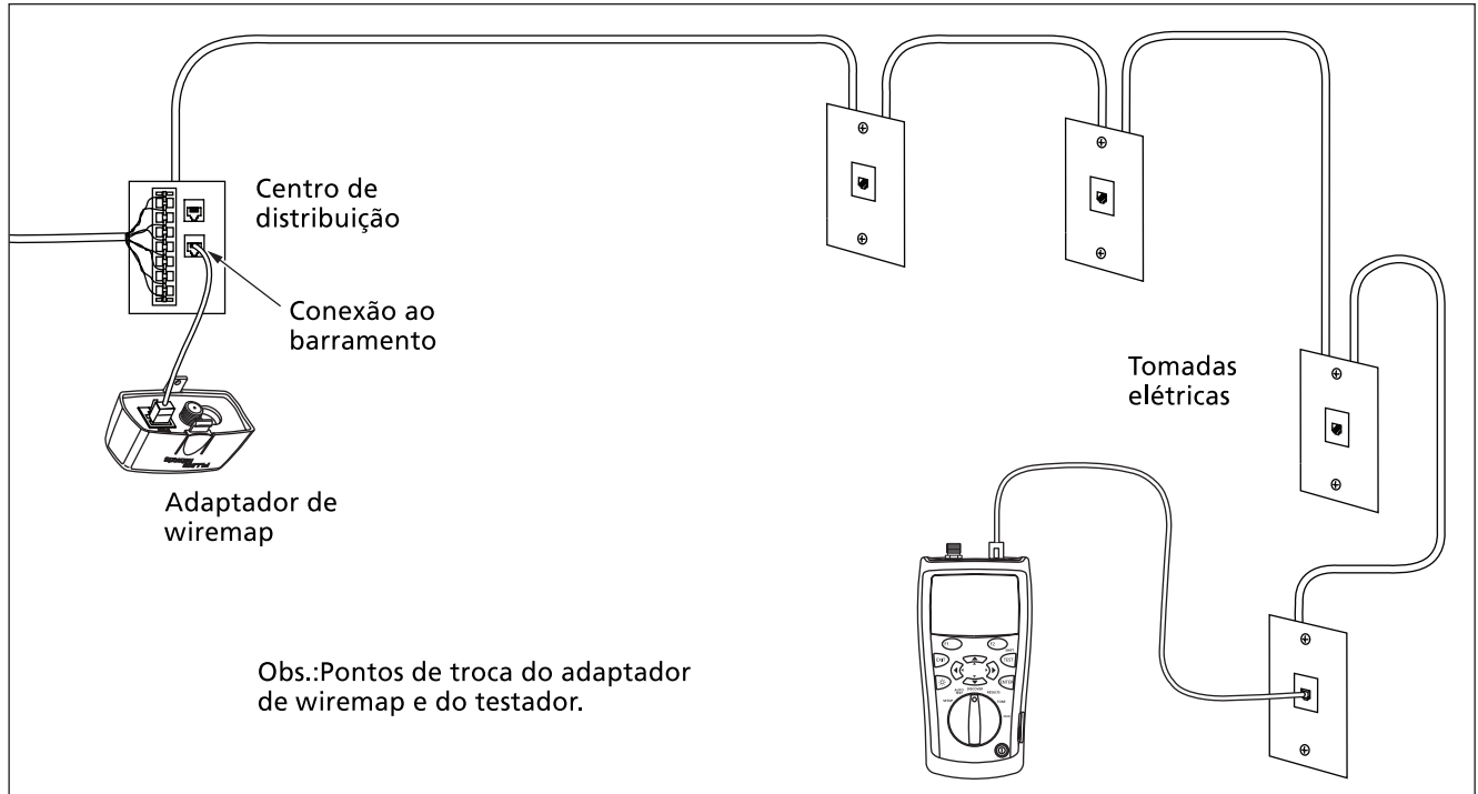
Figura 8. Conexões de Autoteste para cabeamento telefônico com topologia de barramento
