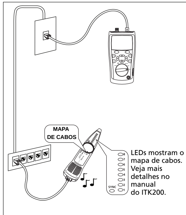
Figura 21. Como usar o gerador de tom com a função de mapa de cabo IP200 IntelliTone
