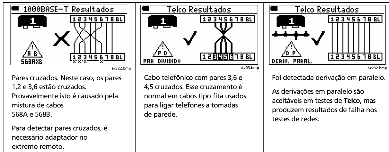
Figura 10. Exibição típica de wiremap (continuação)
