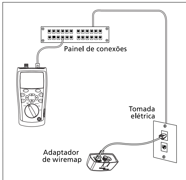
Figura 6. Conexões de Autoteste para cabeamento de rede de par trançado
