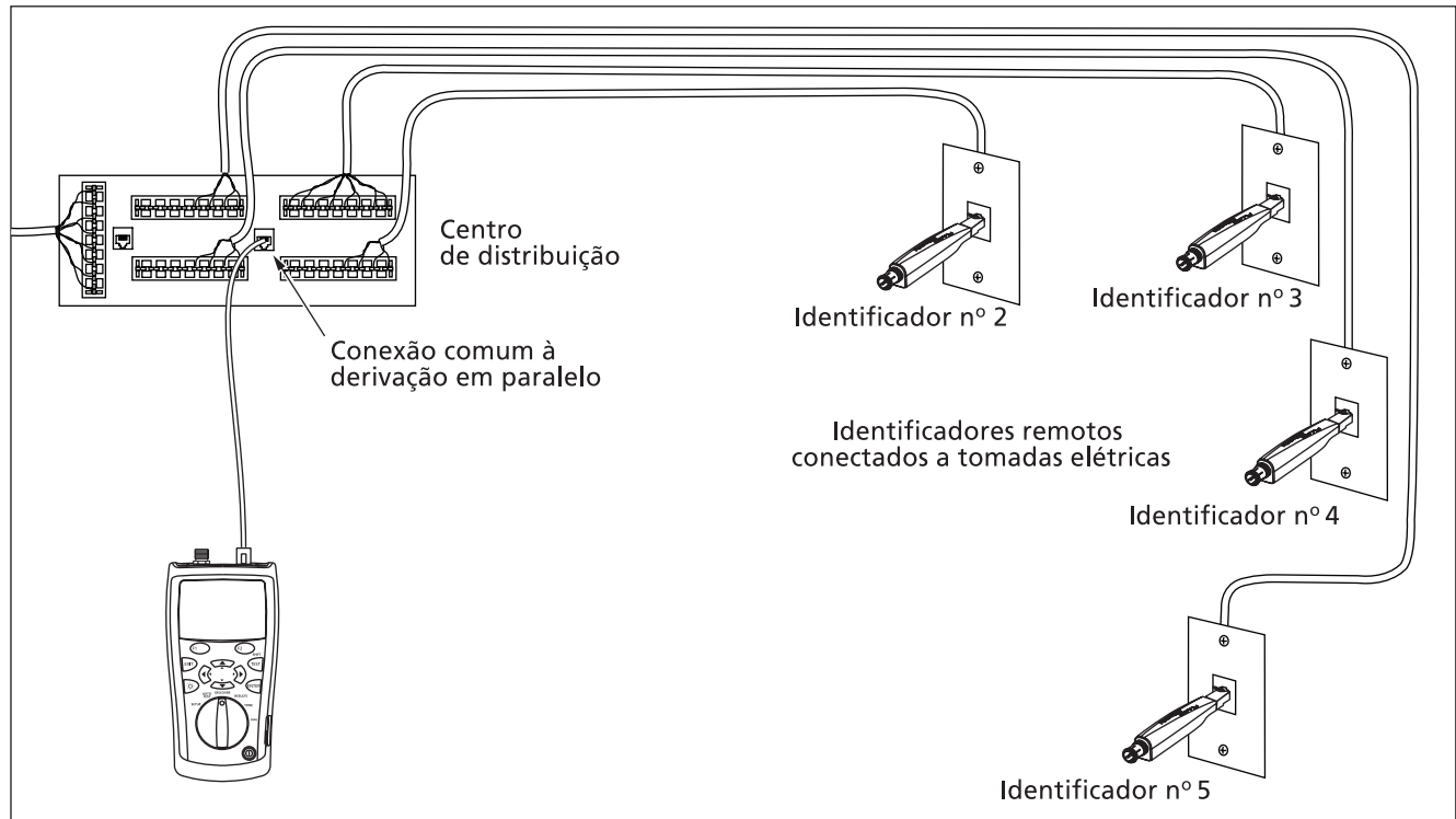
Figura 19. Como usar vários identificadores remotos de cabo
