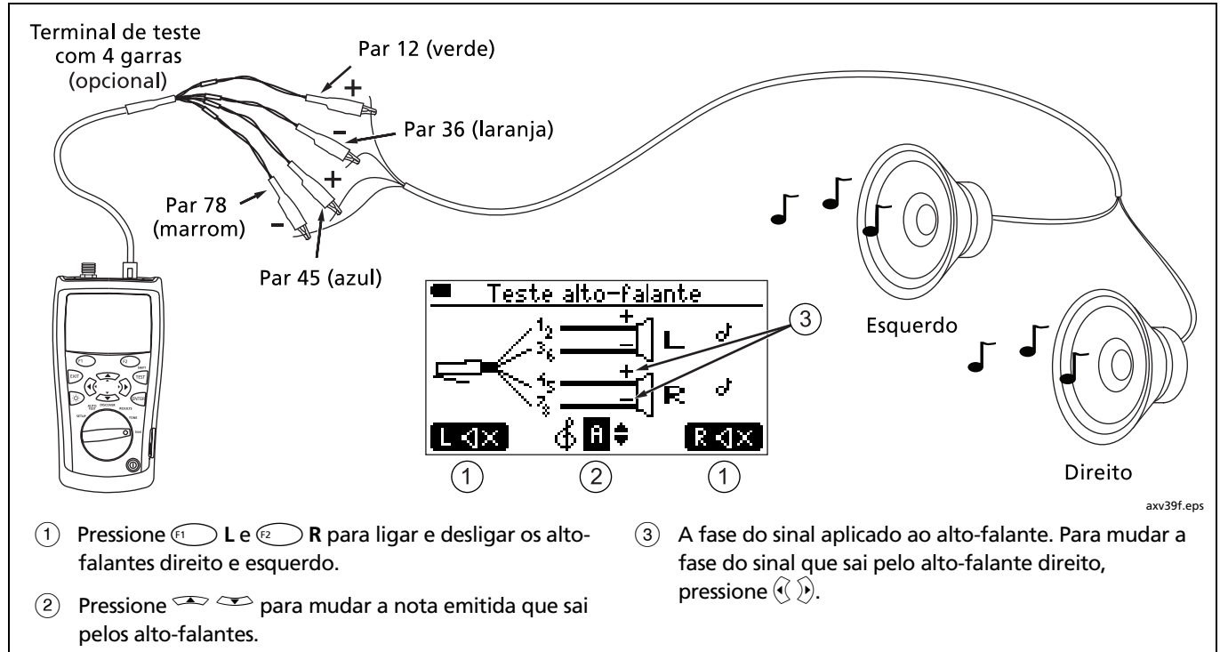
Figura 25. Teste de cabos de alto-falantes
