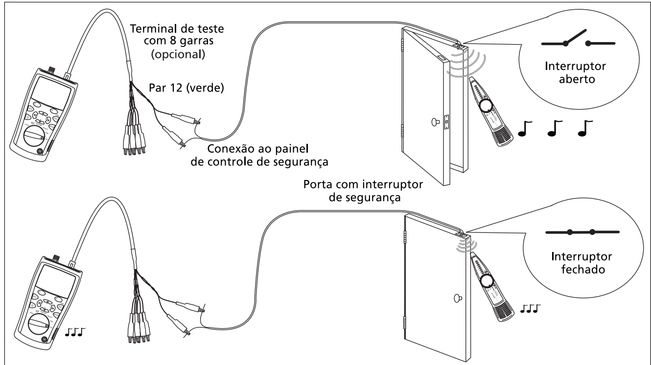
Figura 24. Como usar o gerador de tom de continuidade para testar interruptores de segurança
