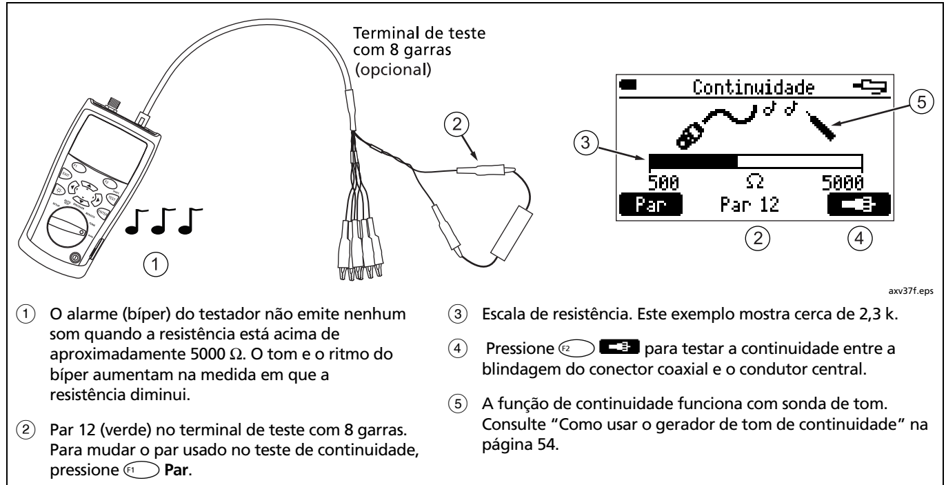
Figura 23. Testes de continuidade
