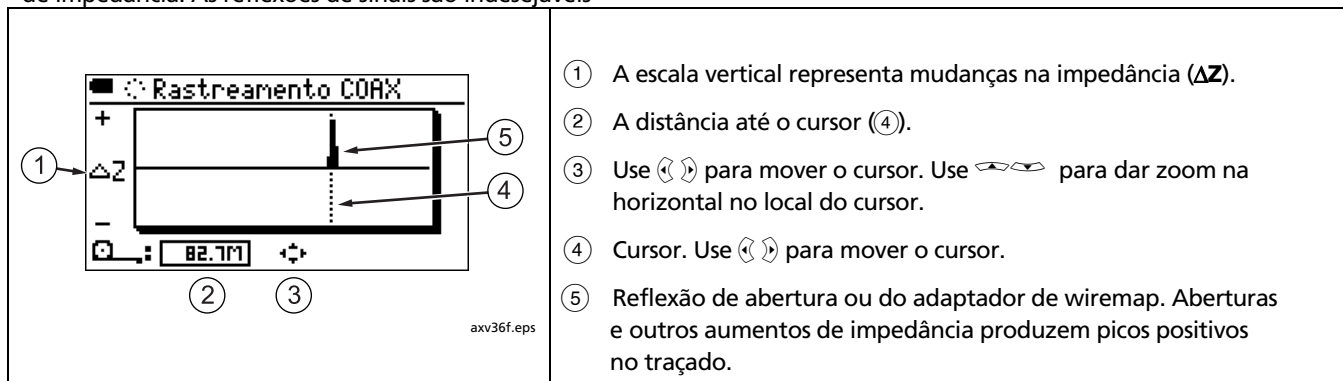
Figura 17. Gráfico de TDR para cabeamento coaxial
