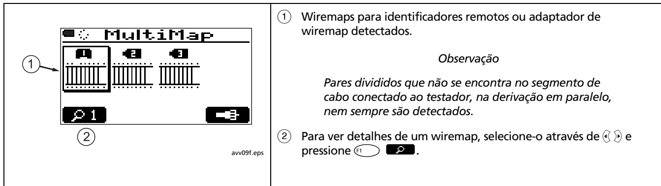
Figura 18. Resultados com a função MultiMap
