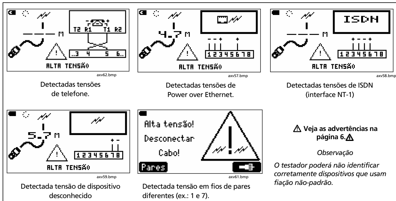
Figura 1. Exemplos de telas de alerta referentes à tensão
