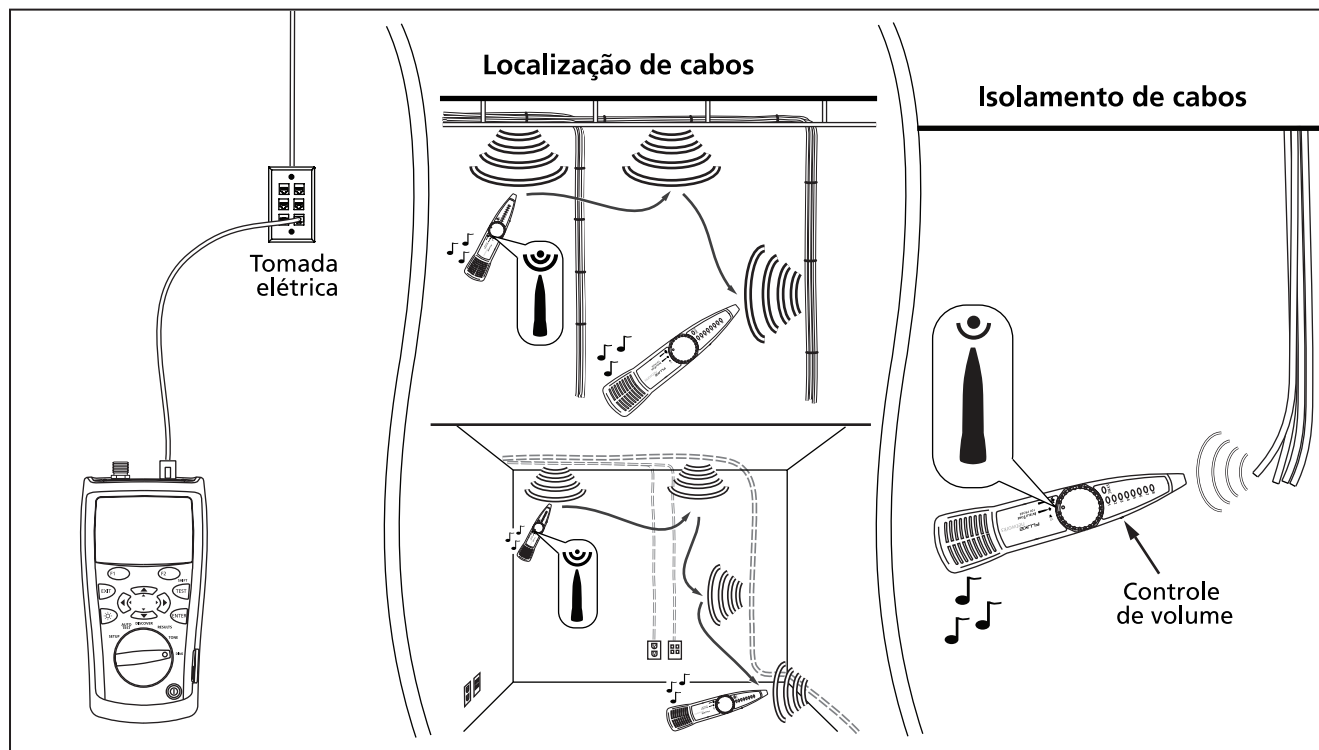
Figura 20. Como usar o gerador de tom (exemplo com par trançado e sonda IntelliTone)
