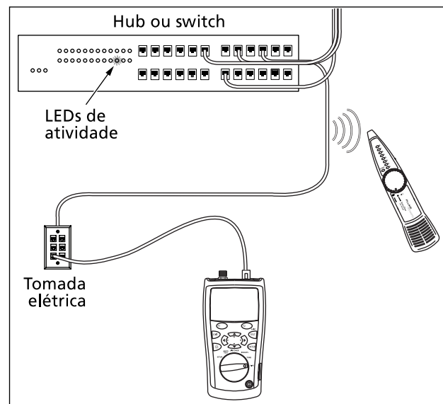
Figura 22. Luz intermitente de porta
