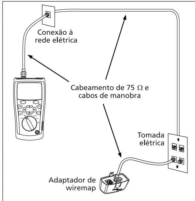
Figura 13. Conexões de Autoteste para cabeamento coaxial
