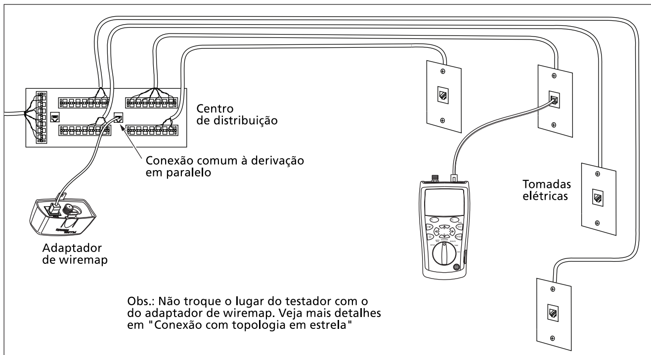
Figura 7. Conexões de Autoteste para cabeamento telefônico com topologia em estrela
