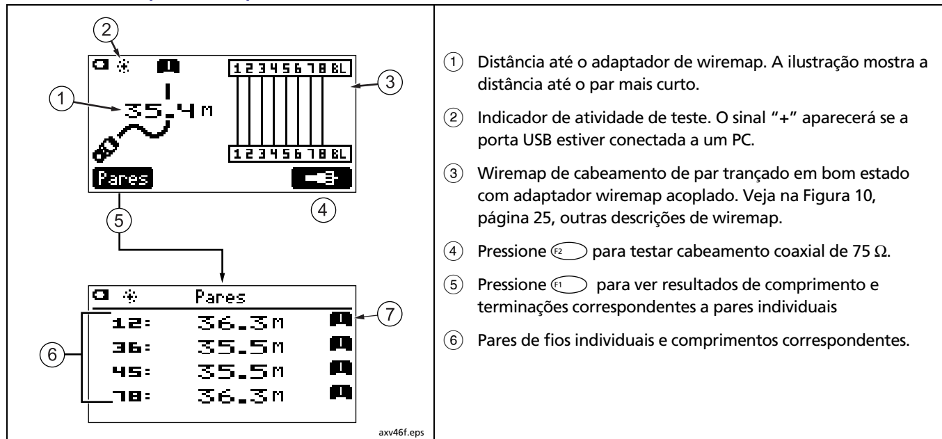
Figura 15. Resultados de cabeamento de par trançado no modo Discover (Descoberta)
