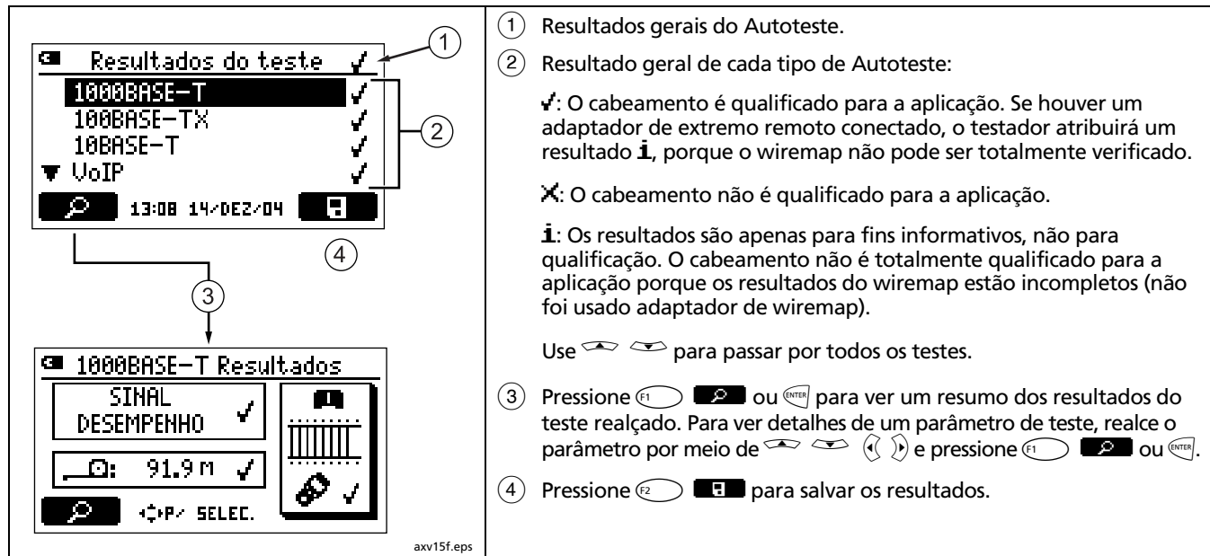
Figura 9. Telas de resumo de Autoteste
