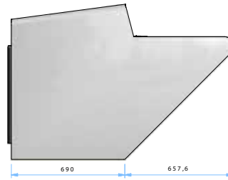
VISTA LATERAL ( 1 : 15 )
